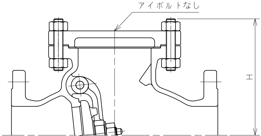
呼び径100・125
