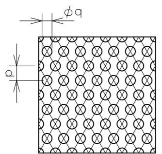
スクリーンのパンチング形態
