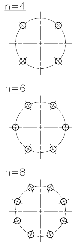
配管フランジ穴位置図
