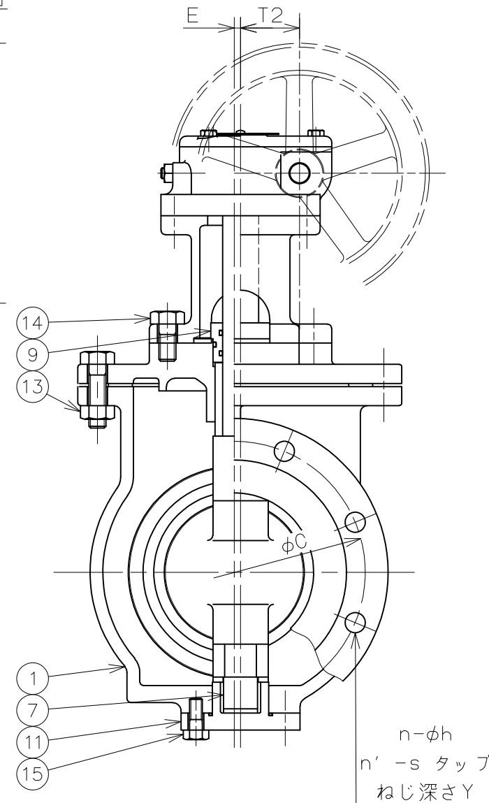
A部: 呼び径75・100
