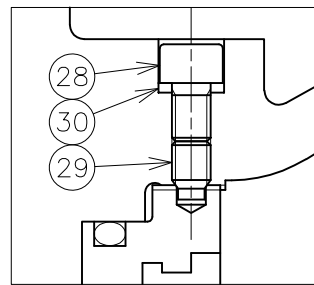
Y部詳細図
