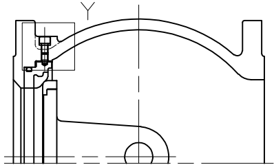
X-X断面図
