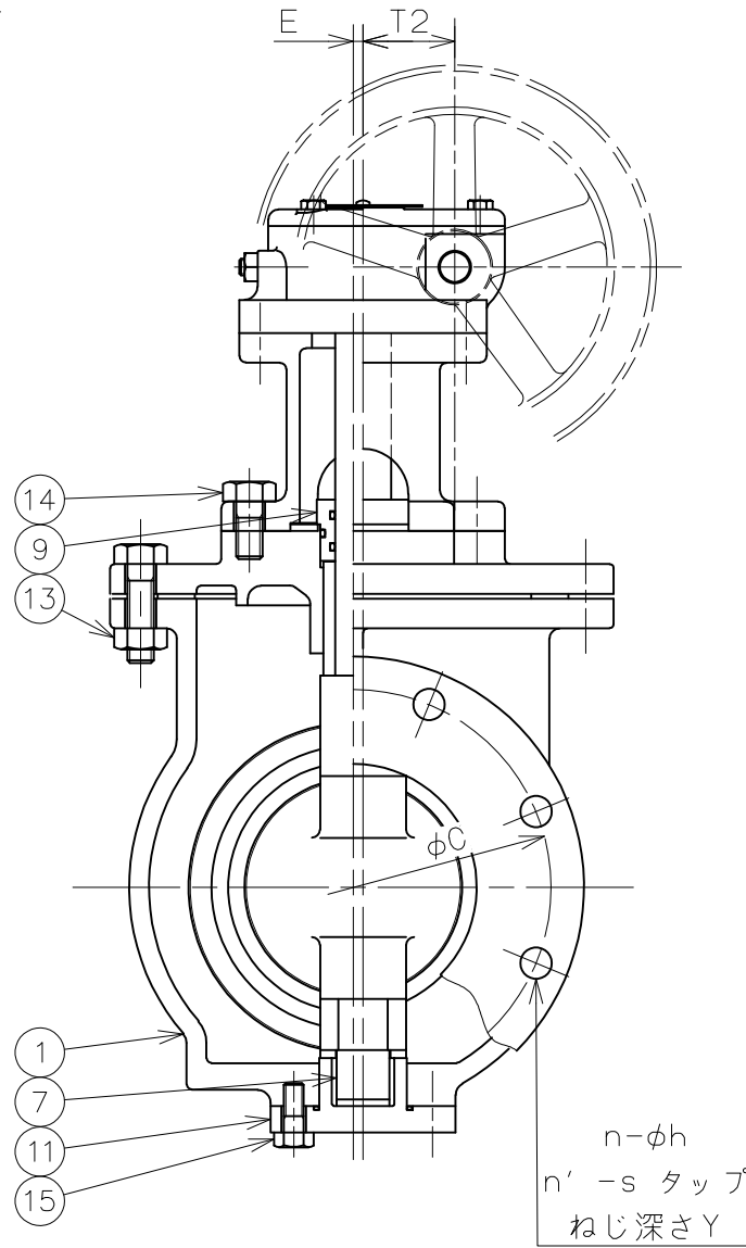
A部: 呼び径80・100
