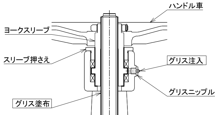
スリーブ部へのグリス注入、塗布例
